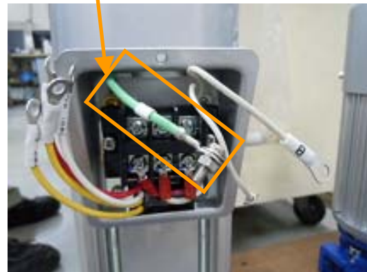
新端子台 新設：アース用リード線（緑色）
