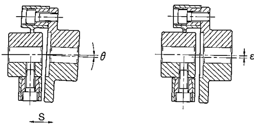
偏心、軸方向変位
